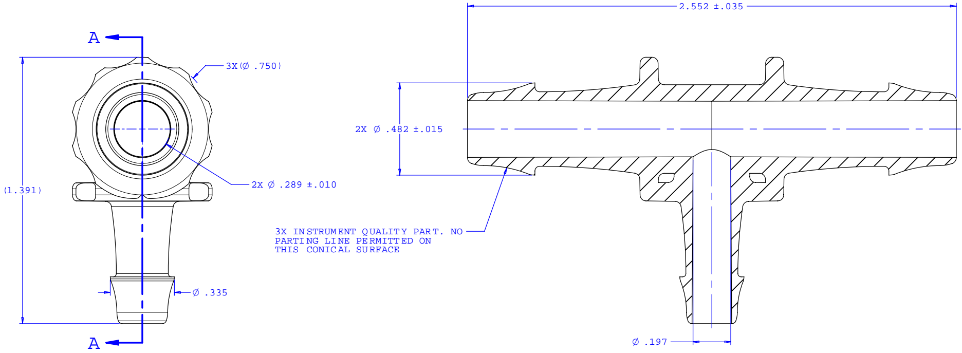
SECTION A-A
